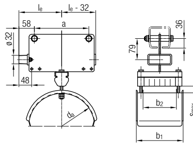
End Clamp 1)
